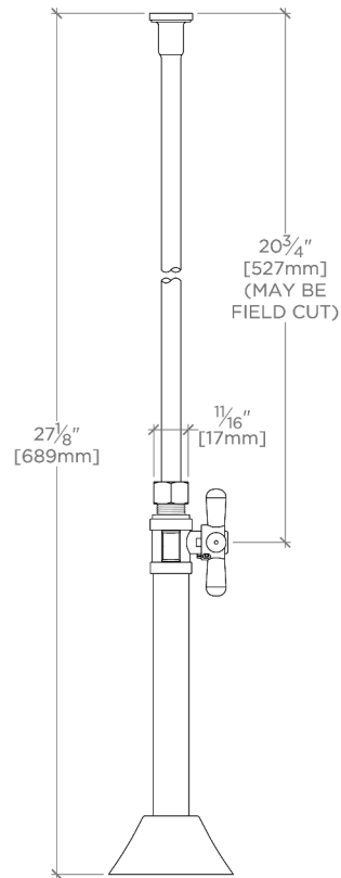
SIDE VIEW SCALE: 3"=1'-0"
