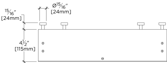
TOP VIEW SCALE: 1 1/2"=1'-0"
