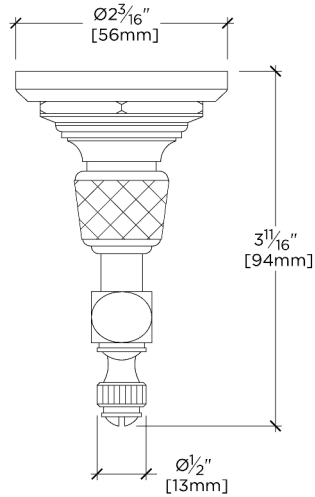
TOP VIEW SCALE: 6"=1'-0"
