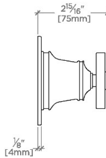
SIDE VIEW SCALE: 3"=1'-0"
