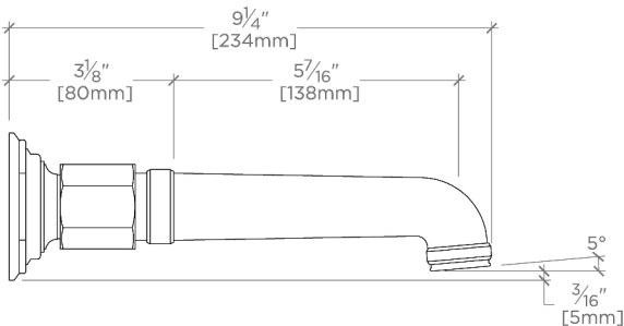
SIDE VIEW SCALE: 3"=1'-0"
