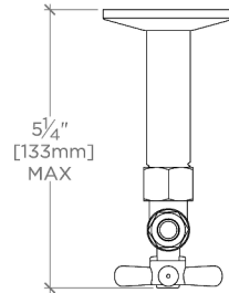
SCALE: 3"=1'-0"
