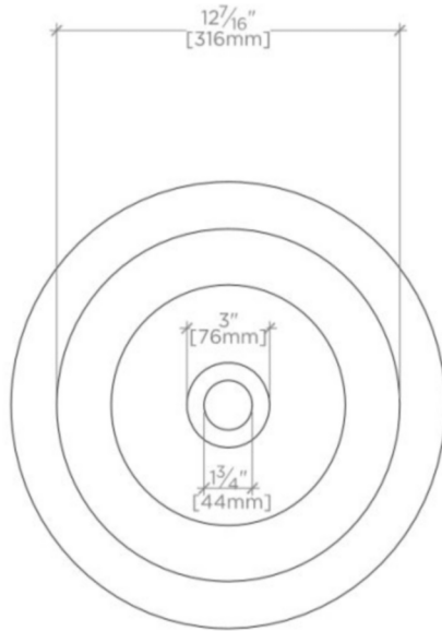
TOP VIEW SCALE: 1 1/2"=1'-0"
