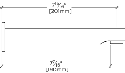
SIDE VIEW SCALE: 3"=1'-0"
