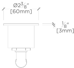
TOP VIEW SCALE: 3"=1'-0"
