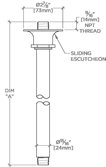
FRONT VIEW SCALE: 3"=1'-0"
