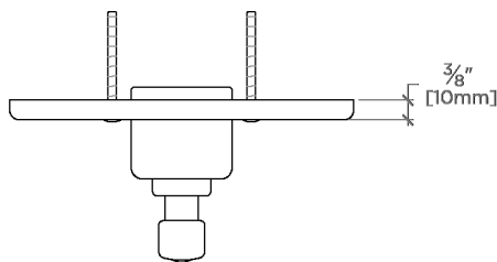
TOP VIEW SCALE: 3"=1'-0"
