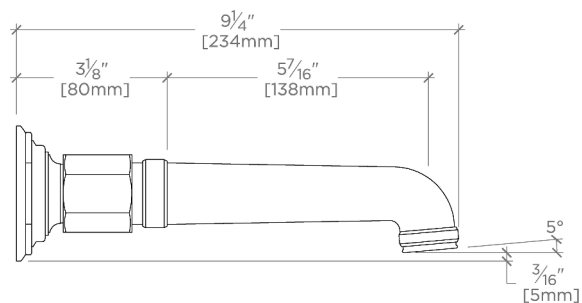
SIDE VIEW SCALE: 3"=1'-0"
