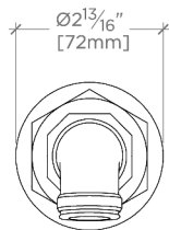
FRONT VIEW SCALE: 3"=1'-0"
