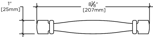
FRONT VIEW SCALE: 3"=1'-0"
