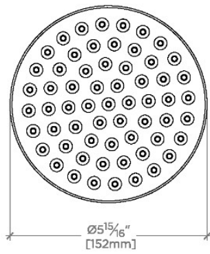
CEILING VIEW SCALE: 3"=1'-0"
