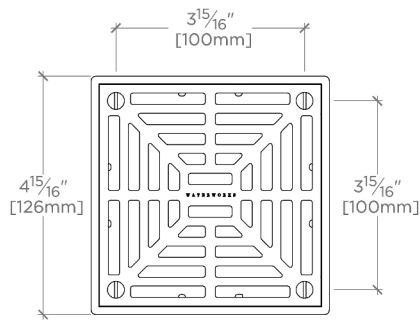
TOP VIEW SCALE: 3"=1'-0"
