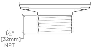
SIDE VIEW SCALE: 3"=1'-0"
