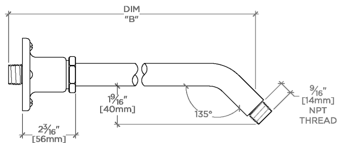
SIDE VIEW SCALE: 3"=1'-0"
