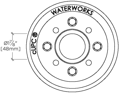
TOP VIEW SCALE: 3"=1'-0"
