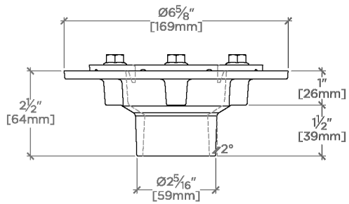
FRONT VIEW SCALE: 3"=1'-0"
