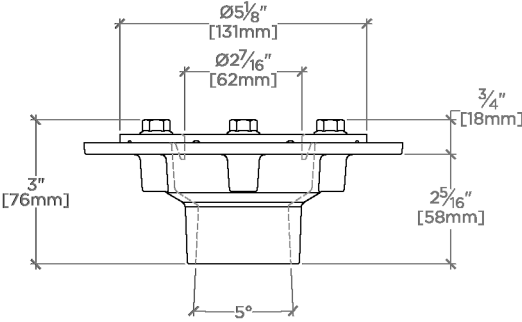
SIDE VIEW SCALE: 3"=1'-0"
