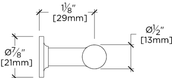
SIDE VIEW SCALE: 6"=1'-0"
