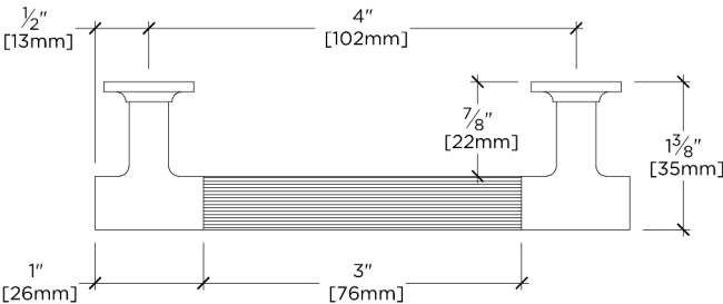
TOP VIEW SCALE: 6"=1'-0"
