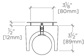
TOP VIEW SCALE: 1 1/2"=1'-0"
