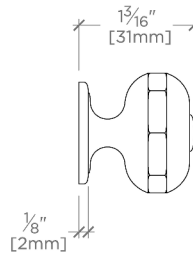
SIDE VIEW SCALE: 6"=1'-0"
