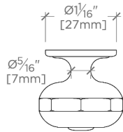
TOP VIEW SCALE: 6"=1'-0"
