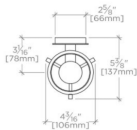
TOP VIEW SCALE: 1/2"=1'-0"
