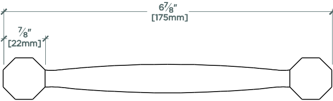
FRONT VIEW SCALE: 6"=1'-0"
