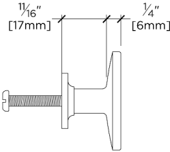
SIDE VIEW SCALE: 6"=1'-0"
