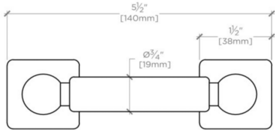
FRONT VIEW SCALE: 6"=1'-0"
