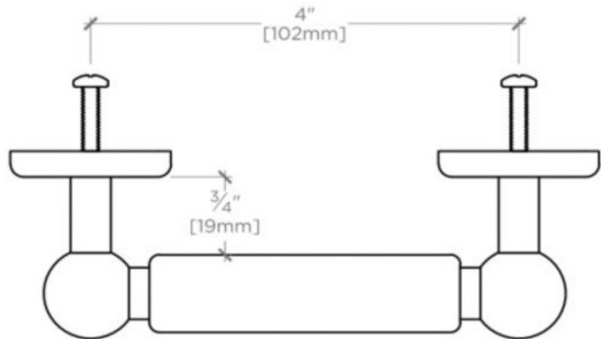
TOP VIEW SCALE: 6"=1'-0"
