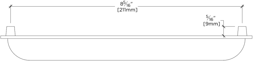
TOP VIEW SCALE: 6"=1'-0"
