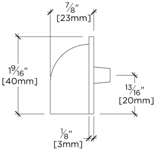
SIDE VIEW SCALE: 6"=1'-0"
