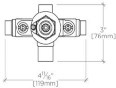
FRONT VIEW SCALE: 3"=1'-0"
