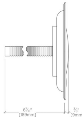
SIDE VIEW SCALE: 3"=1'-0"
