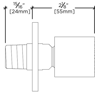
SIDE VIEW SCALE: 6"=1'-0"
