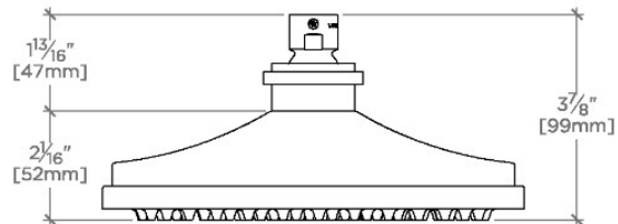
SIDE VIEW SCALE: 3"=1'-0"
