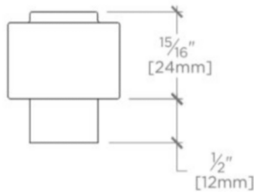
FRONT VIEW SCALE: 6"=1'-0"
