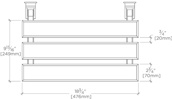
TOP VIEW SCALE: 1 1/2" = 1'-0"
