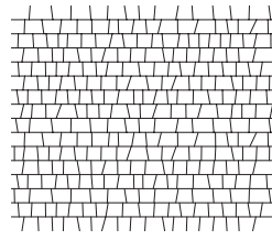
1.5cm HANDCLIPPED (KSSMHC)
