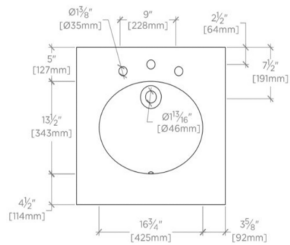
TOP VIEW SCALE: 3/4"=1'-0"
