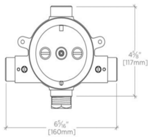
FRONT VIEW SCALE: 3"=1'-0"
