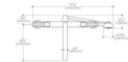
TOP VIEW SCALE: 3/4"=1'-0"
