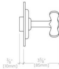
SIDE VIEW SCALE: 3"=1'-0"
