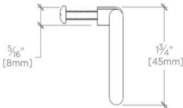
SIDE VIEW SCALE: 6"=1'-0"
