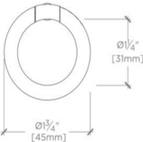
FRONT VIEW SCALE: 6"=1'-0"
