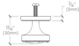
TOP VIEW SCALE: 6"=1'-0"
