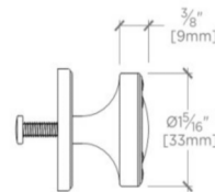
SIDE VIEW SCALE: 6"=1'-0"
