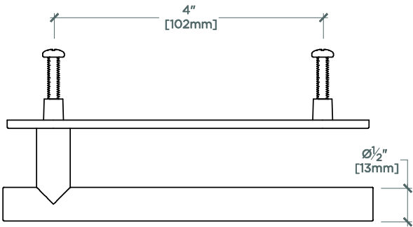
TOP VIEW SCALE: 6"=1'-0"
