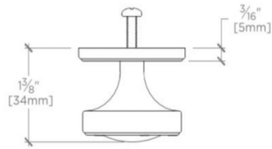
TOP VIEW SCALE: 6"=1'-0"
