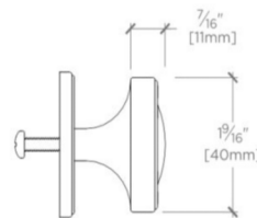
SIDE VIEW SCALE: 6"=1'-0"
