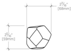
FRONT VIEW SCALE: 3"=1'-0"
