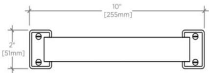
FRONT VIEW SCALE: 3"=1'-0"
