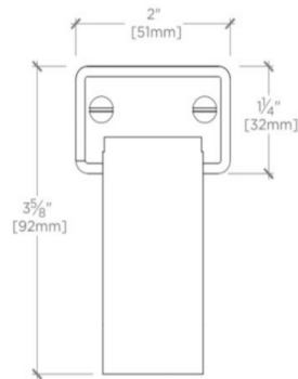
FRONT VIEW SCALE: 6"=1'-0"
