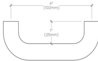
TOP VIEW SCALE: 6"=1'-0"
