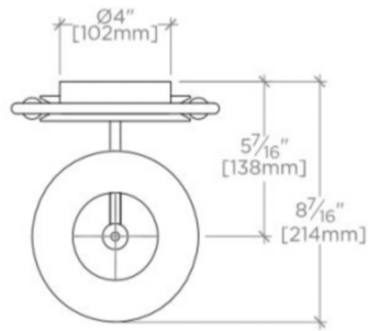
TOP VIEW SCALE: 1 1/2"=1'-0"
