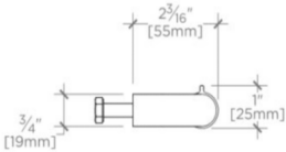
SIDE VIEW SCALE: 3"=1'-0"
