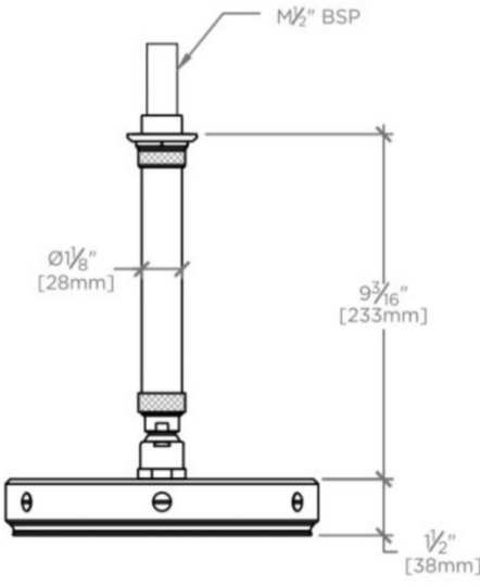
SIDE VIEW SCALE: 2"=1'-0"
