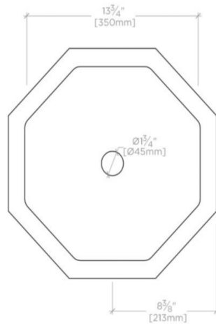
TOP VIEW SCALE: 1/2"=1'-0"
