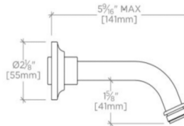
SIDE VIEW SCALE: 3"=1'-0"
